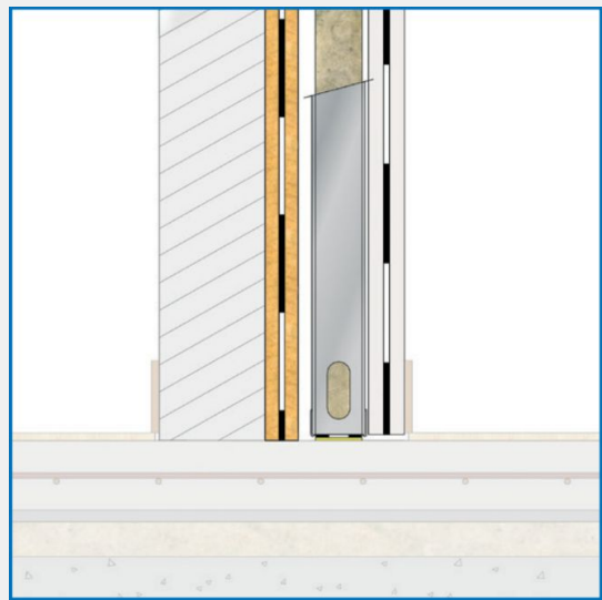
Secțiune pardoseală
