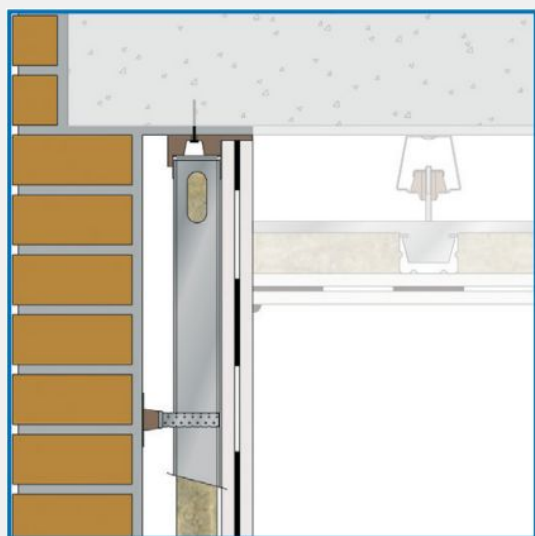
Secțiune tavan
