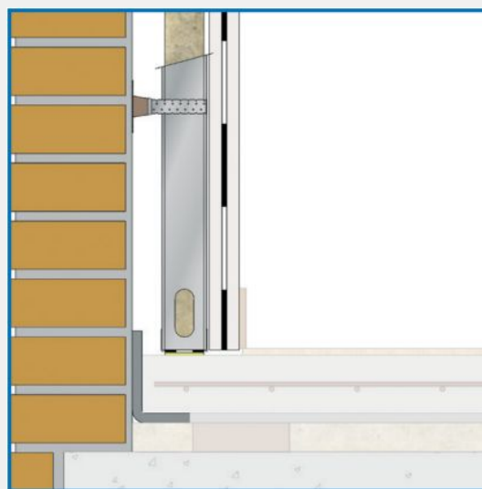
Secțiune pardoseala
